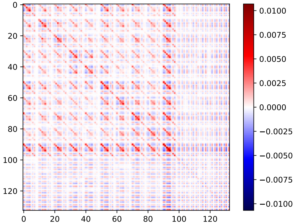
Hesse-Matrix für n = 10
